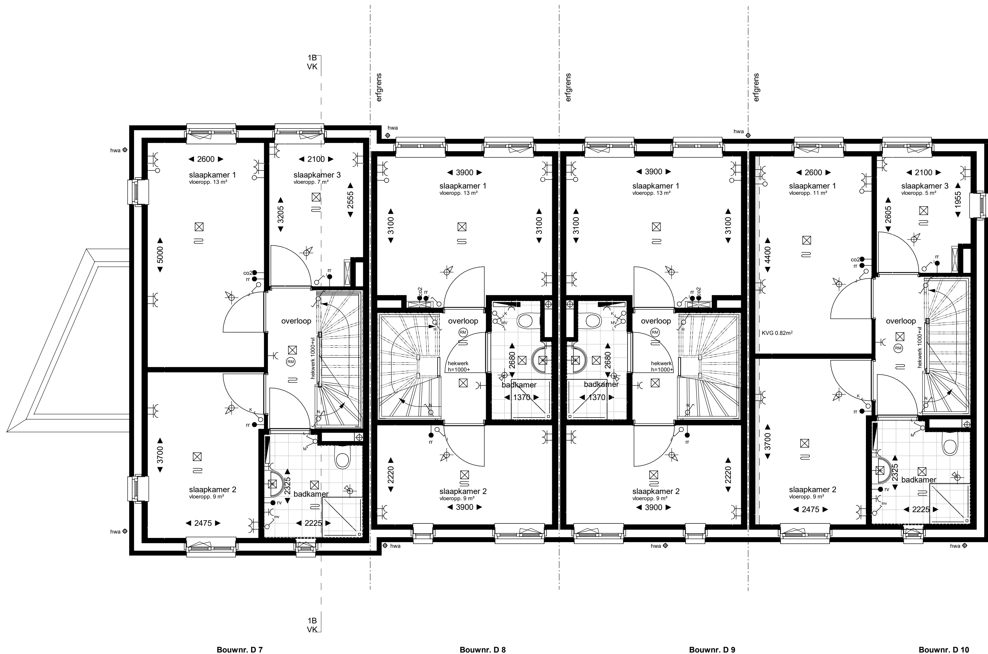
eerste verdieping 1 : 50
