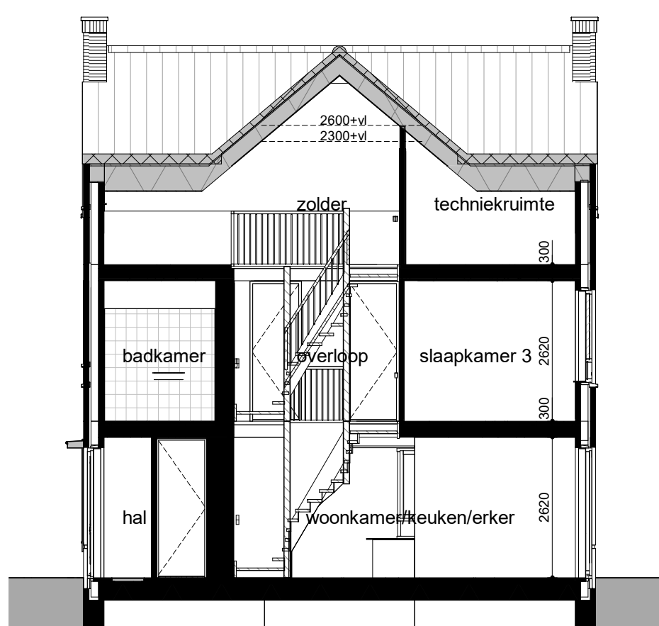
Bouwnr. D 7 doorsnede AA 1 : 100
