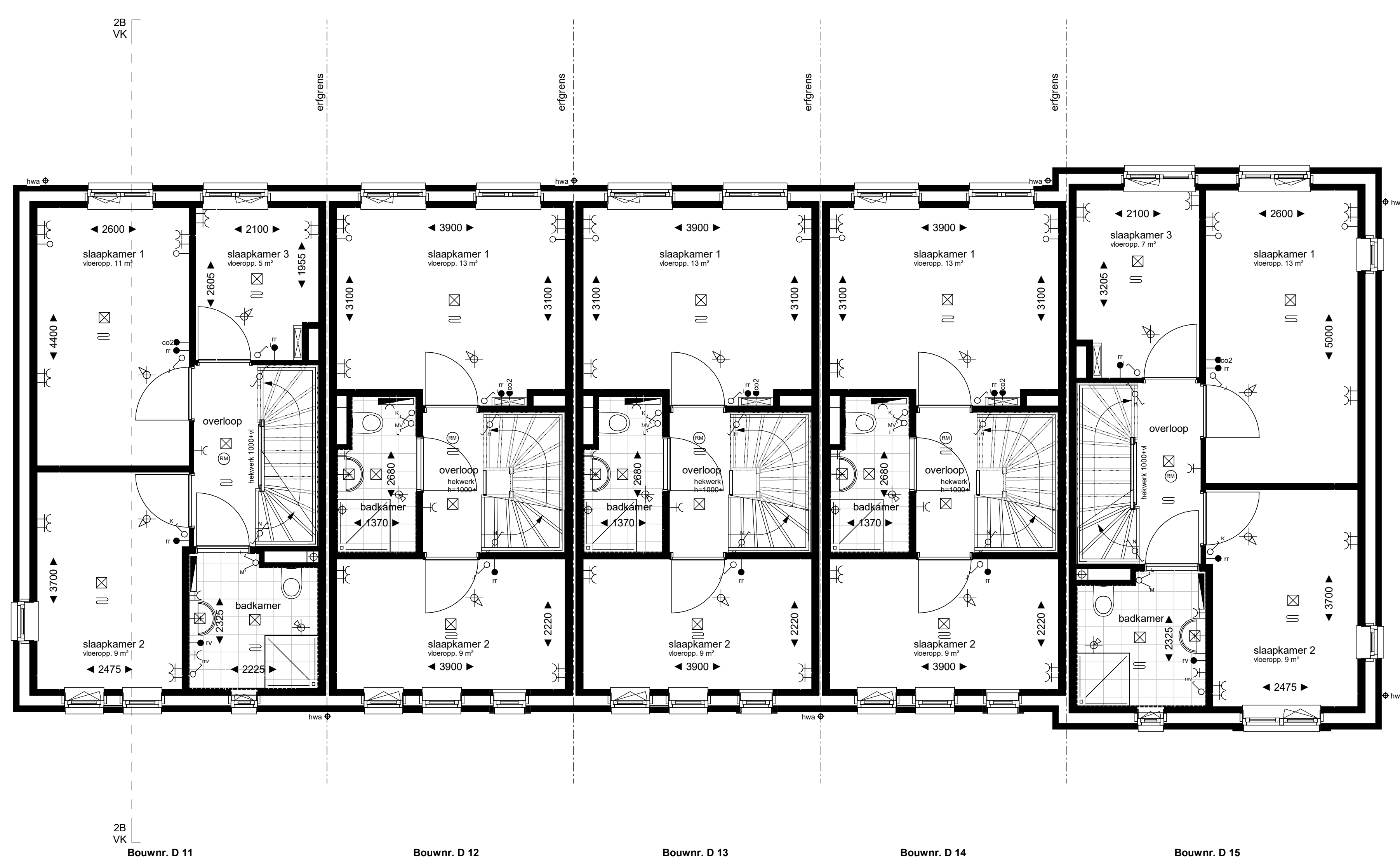
eerste verdieping 1:50
