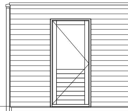
Achtergevel (1:50)
