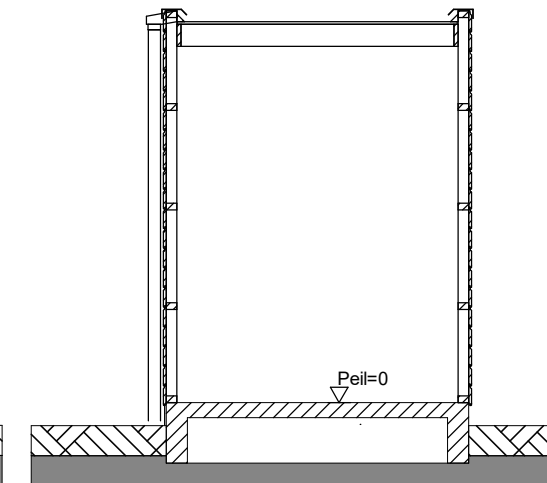
Doorsnede (1:50)
