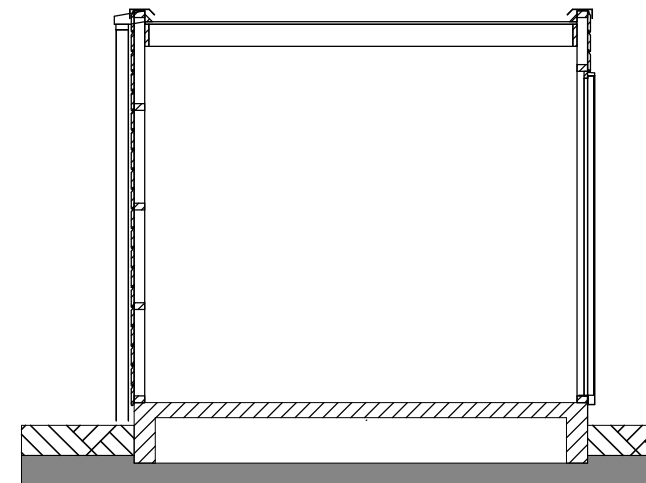
Doorsnede (1:50)
