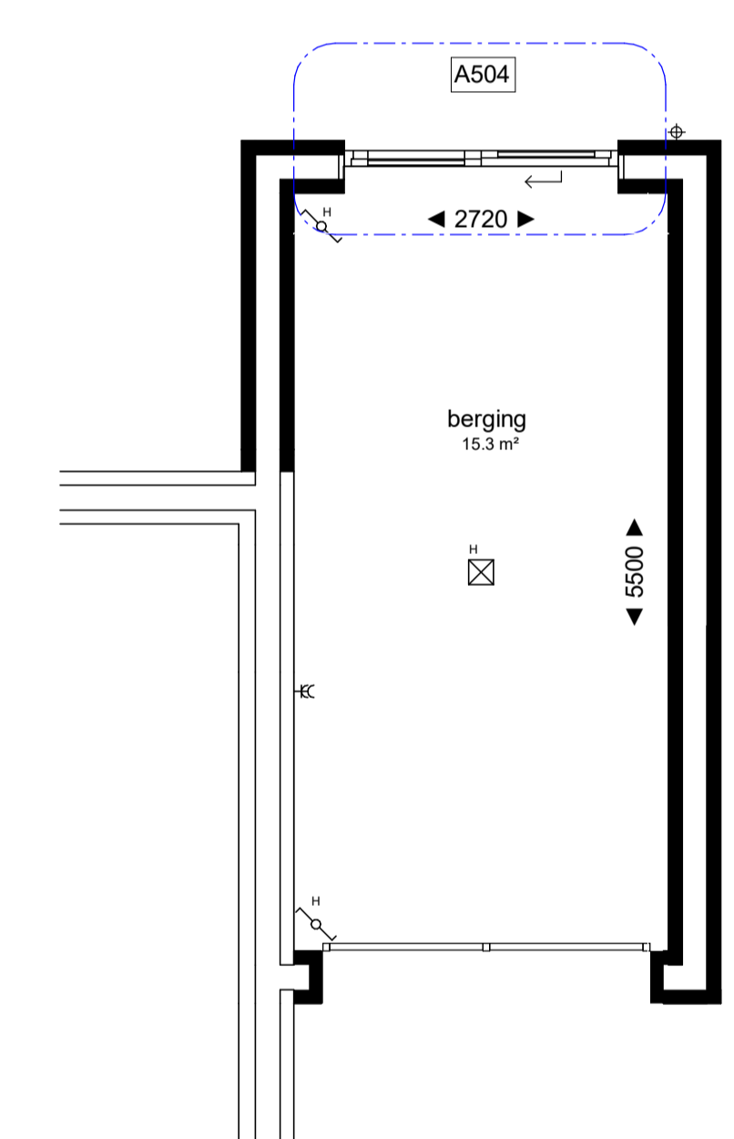
optie: A504 als getekend bwnr(s): D 10, D 20 en H 15 als gespiegeld bwnr(s): D11, D21 en H26
