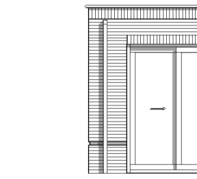
optie: A504 get. bwnrs: D10, D20 en H15 gesp.: bwnrs: D11 en H26 bwnrs: D11, H15 en H26 zonder terugliggende laag / plint
