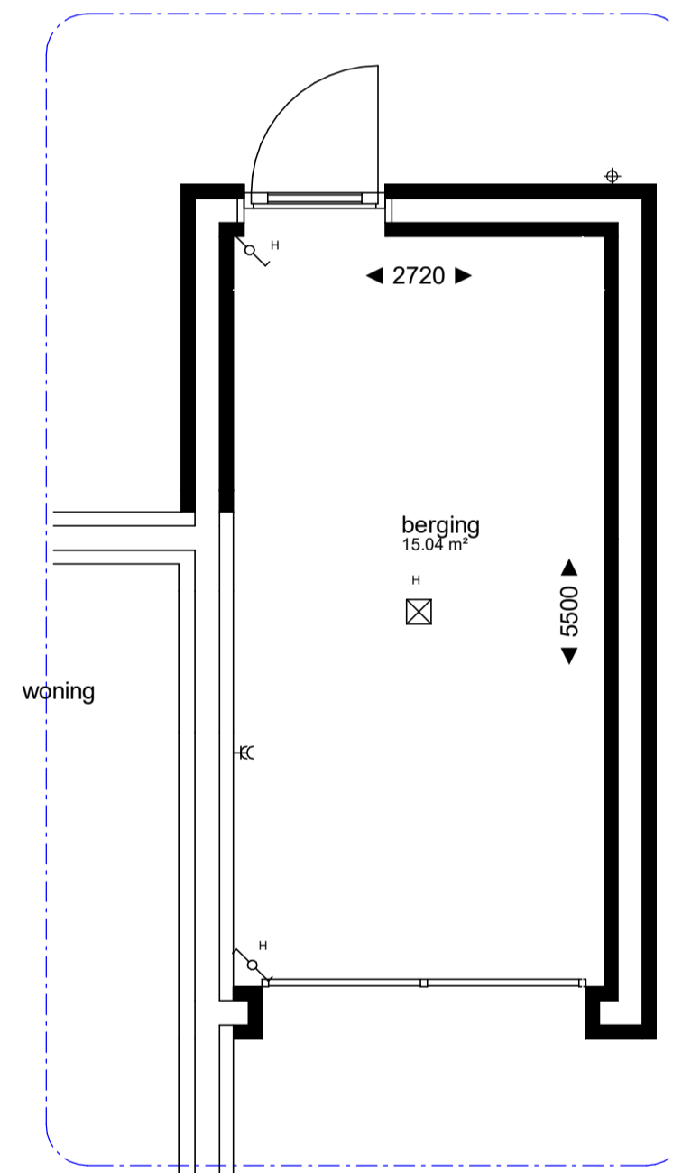
optie: A073A als getekend bwnr(s): D 10, D 20 en H 15 als gespiegeld bwnr(s): D11, D21 en H26
