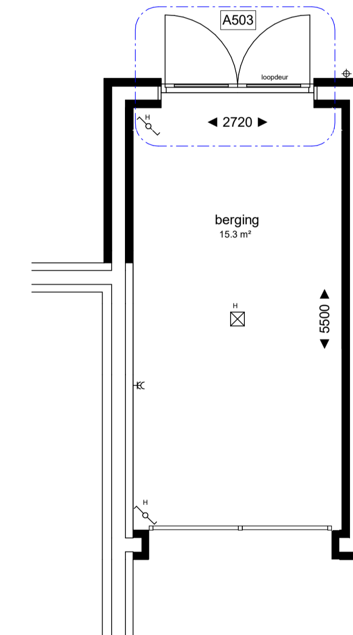
optie: A503 als getekend bwnr(s): D 10, D 20 en H 15 als gespiegeld bwnr(s): D11, D21 en H26
