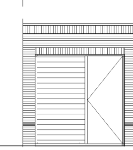
optie: A082 get. bwnrs: D10, D20 en H15 gesp.: bwnrs: D11 en H26 bwnrs: D11, H15 en H26 zonder terugliggende laag / plint
