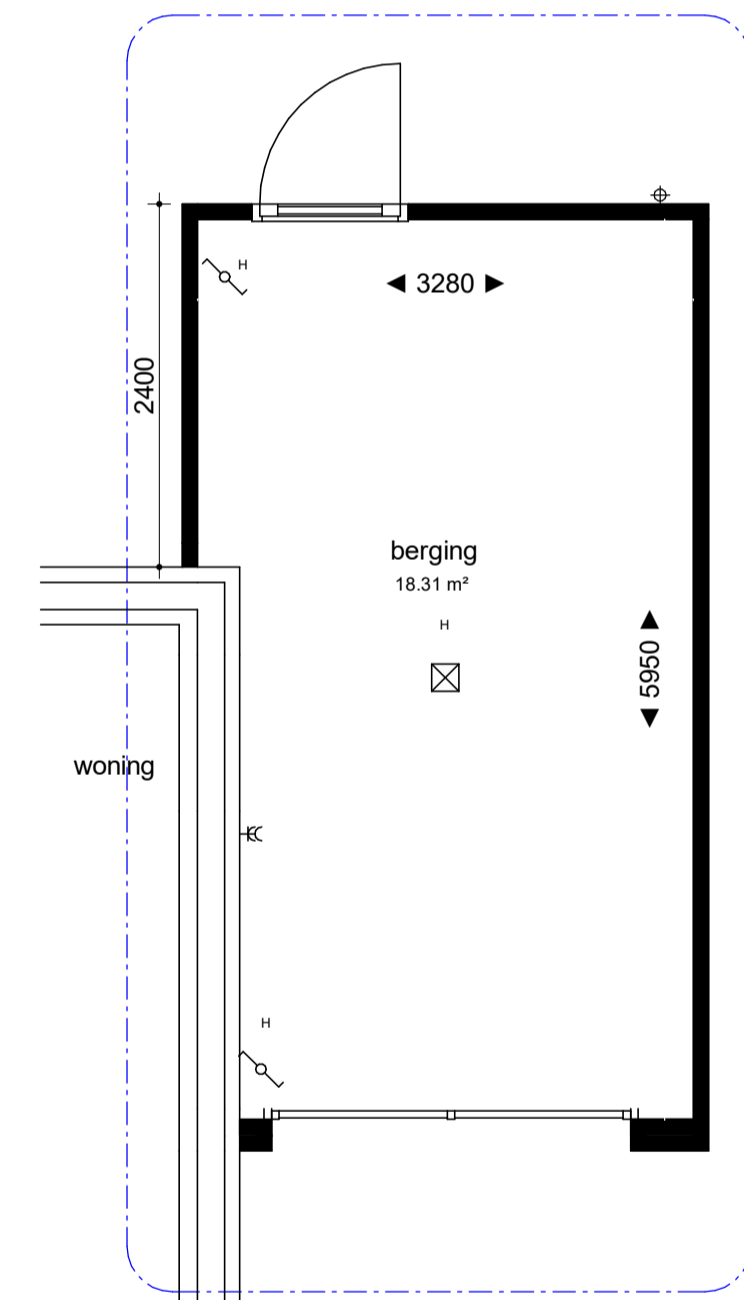
optie: A072A als getekend bwnr(s): D 10, D 20 en H 15 als gespiegeld bwnr(s): D11, D21 en H26
