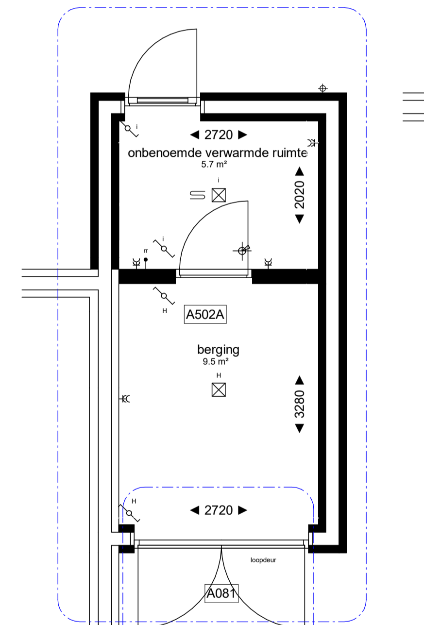
optie: A502A / A081 als getekend bwnr(s): D 10, D 20 en H 15 als gespiegeld bwnr(s): D11, D21 en H26
