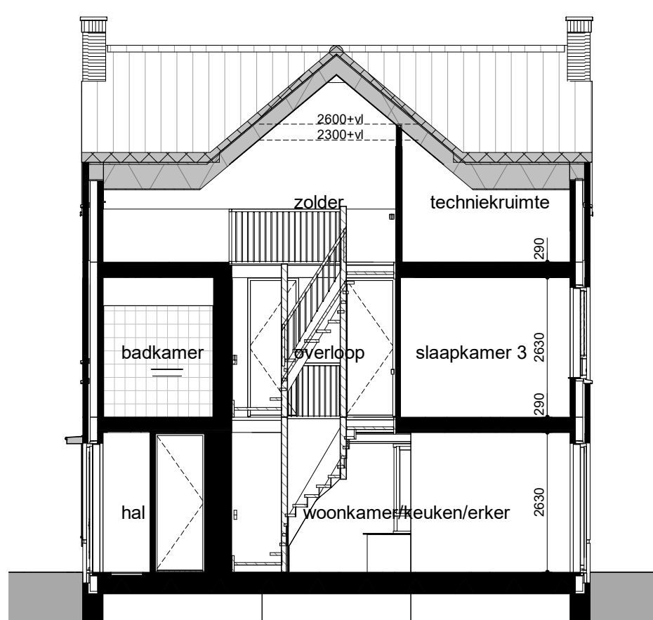
doorsnede AA 1:100
