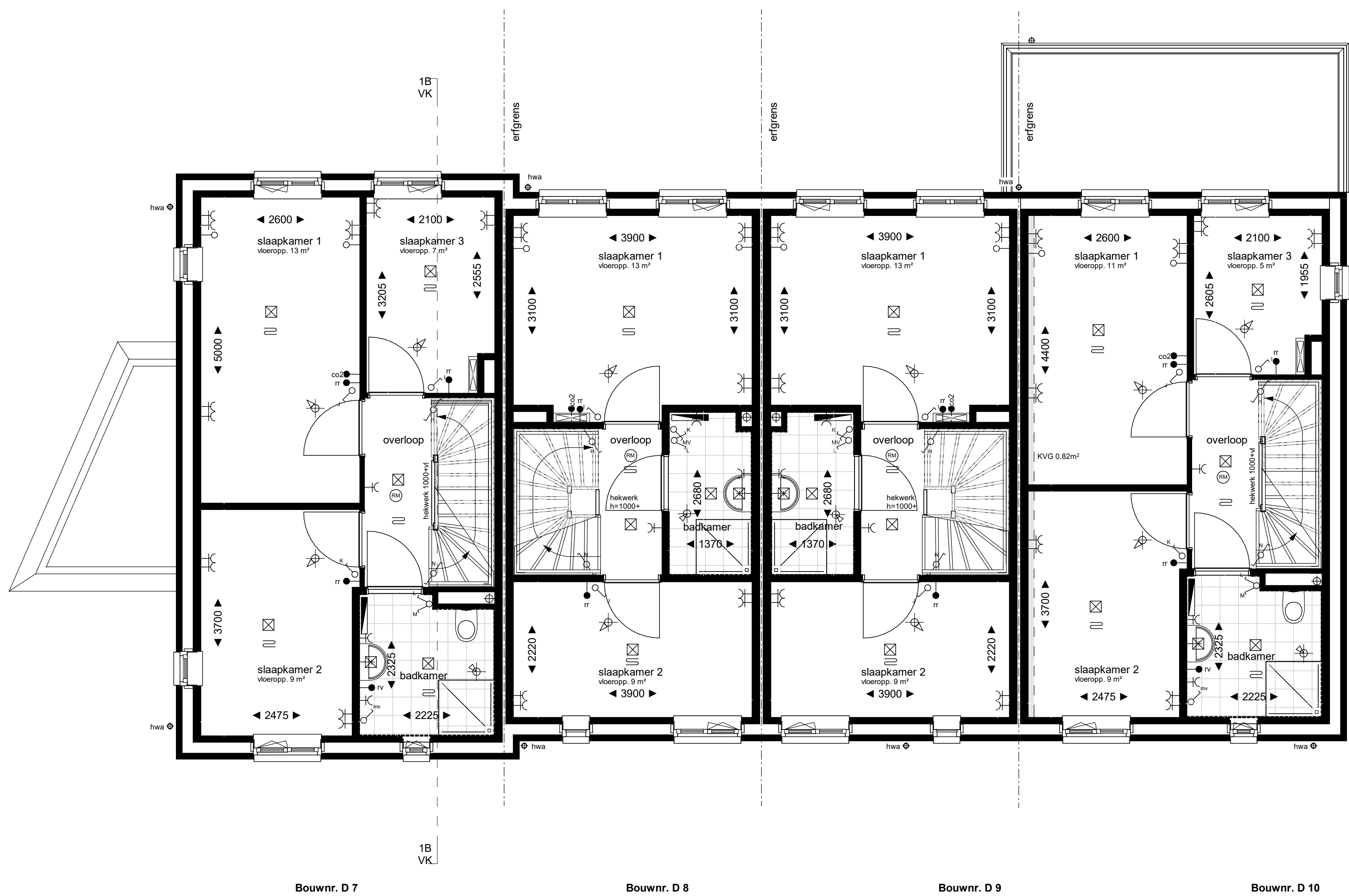
eerste verdieping 1 : 50
