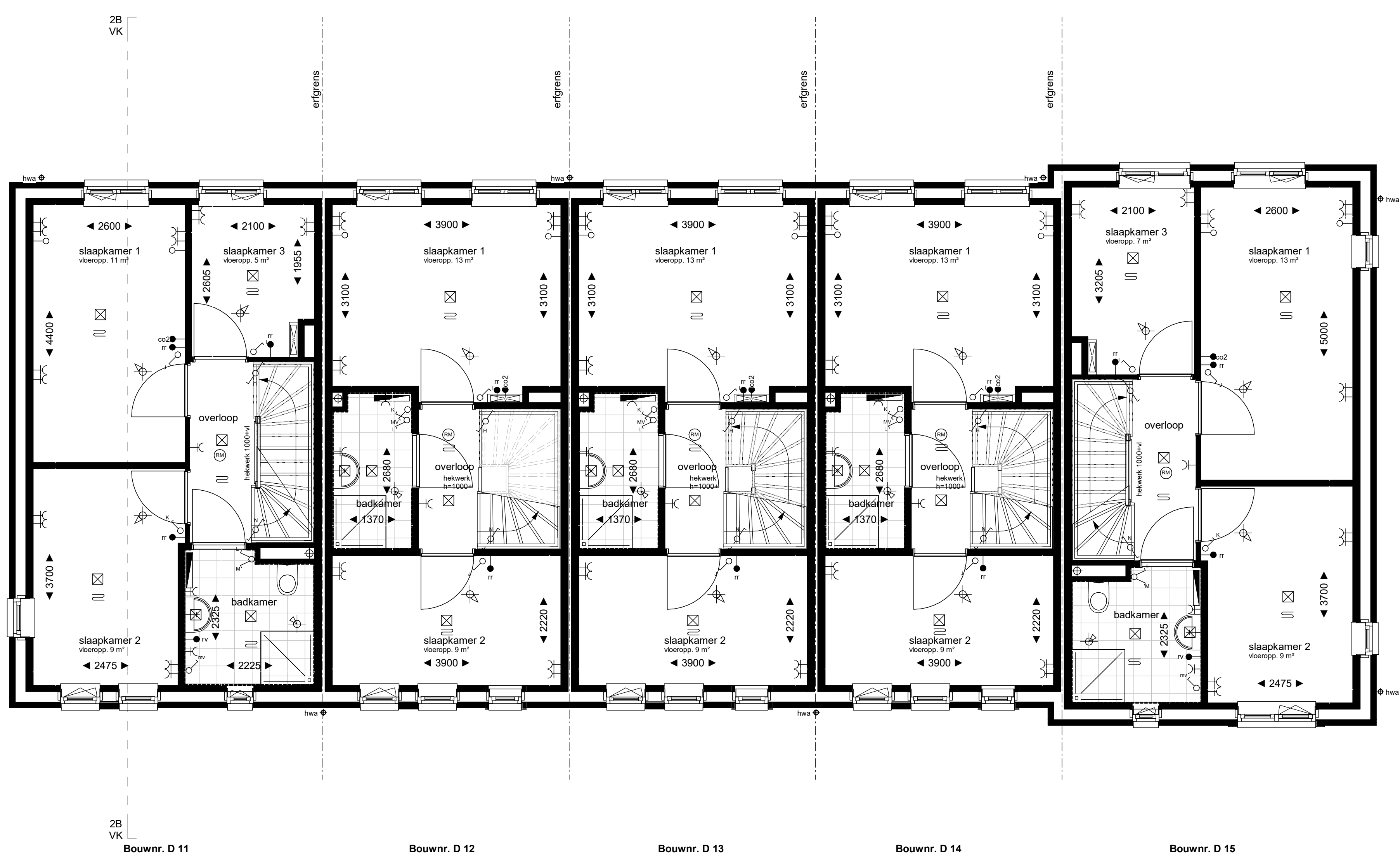
eerste verdieping 1:50
