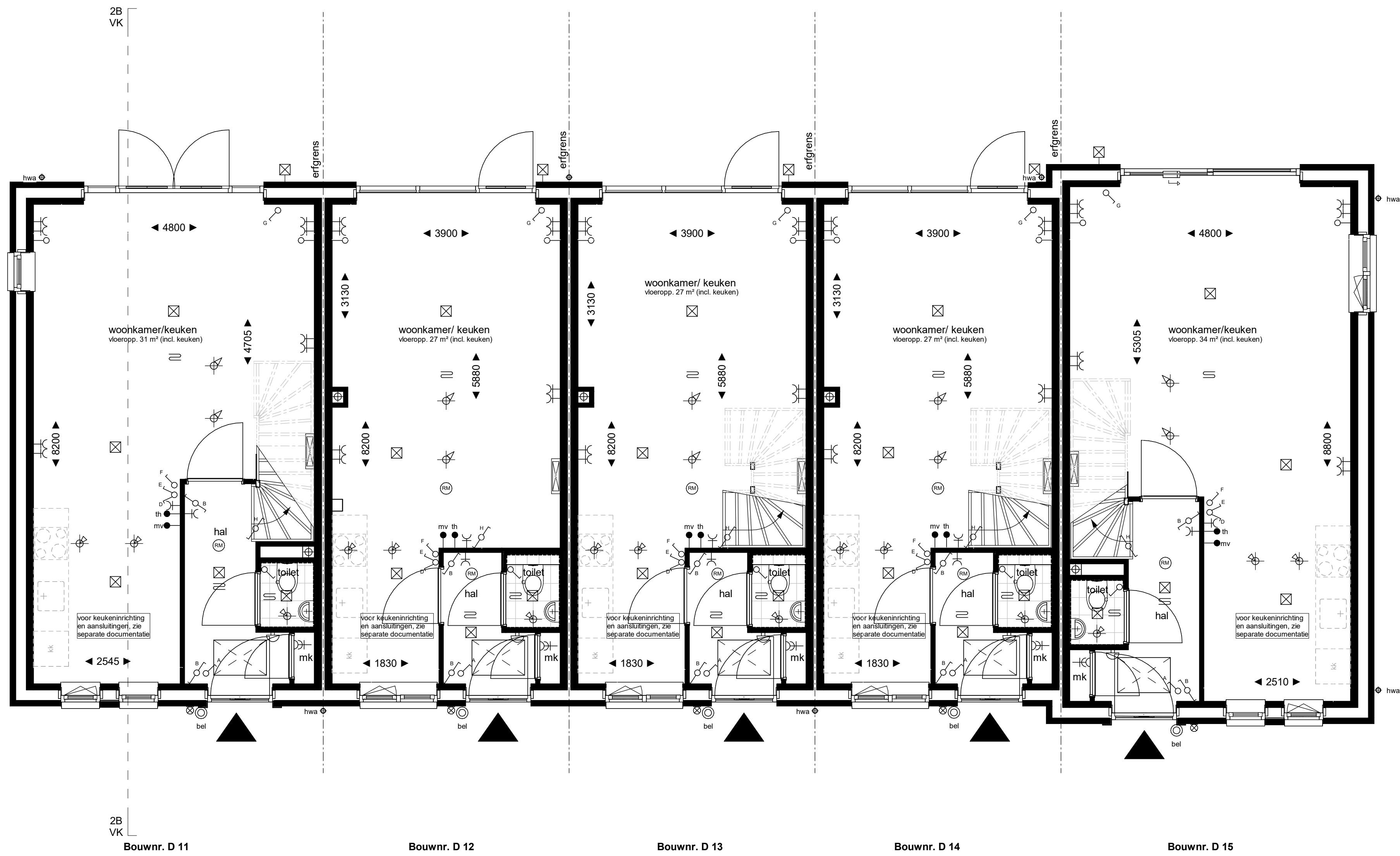
begane grond 1:50
