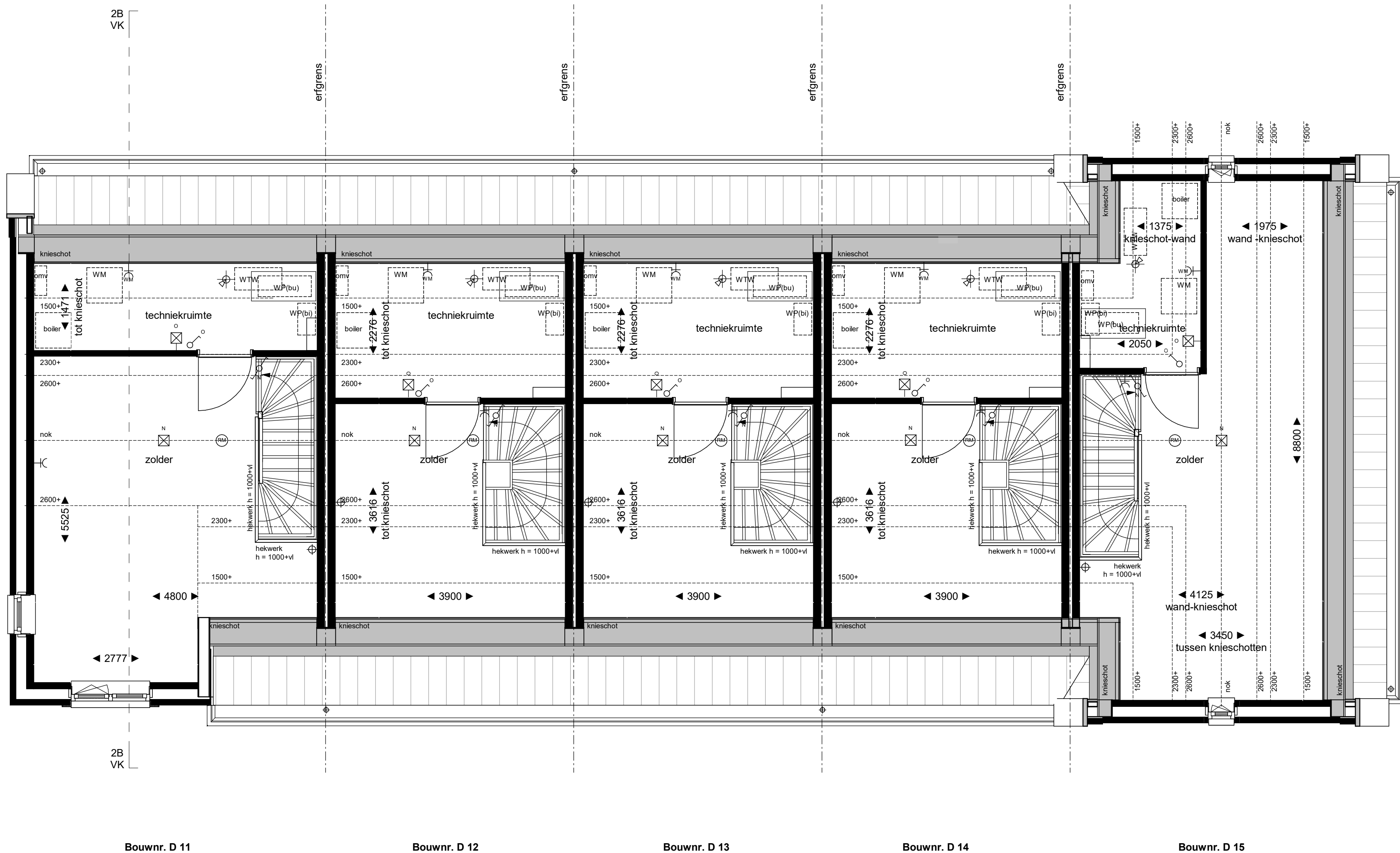
tweede verdieping 1:50
