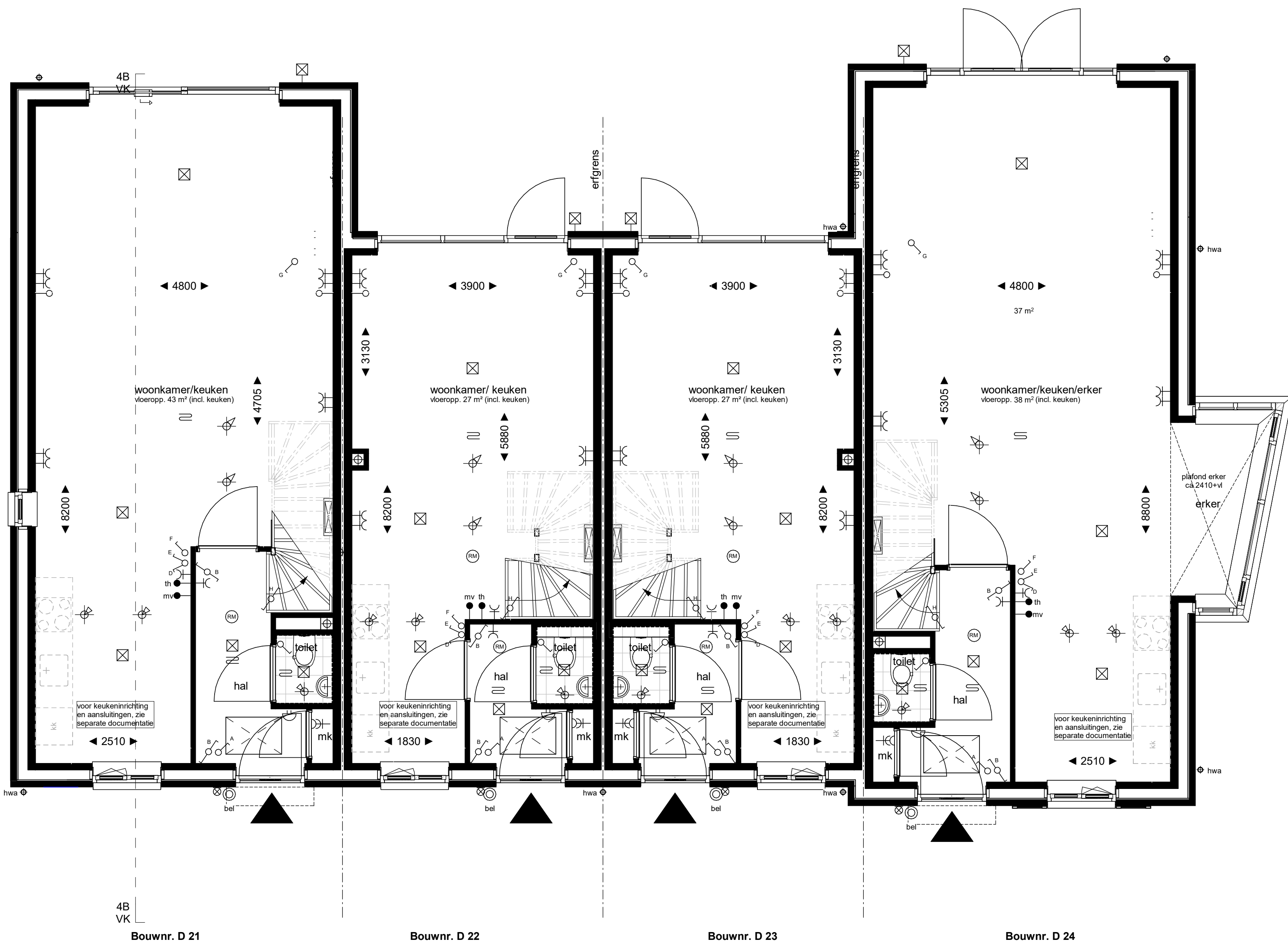
begane grond 1:50
