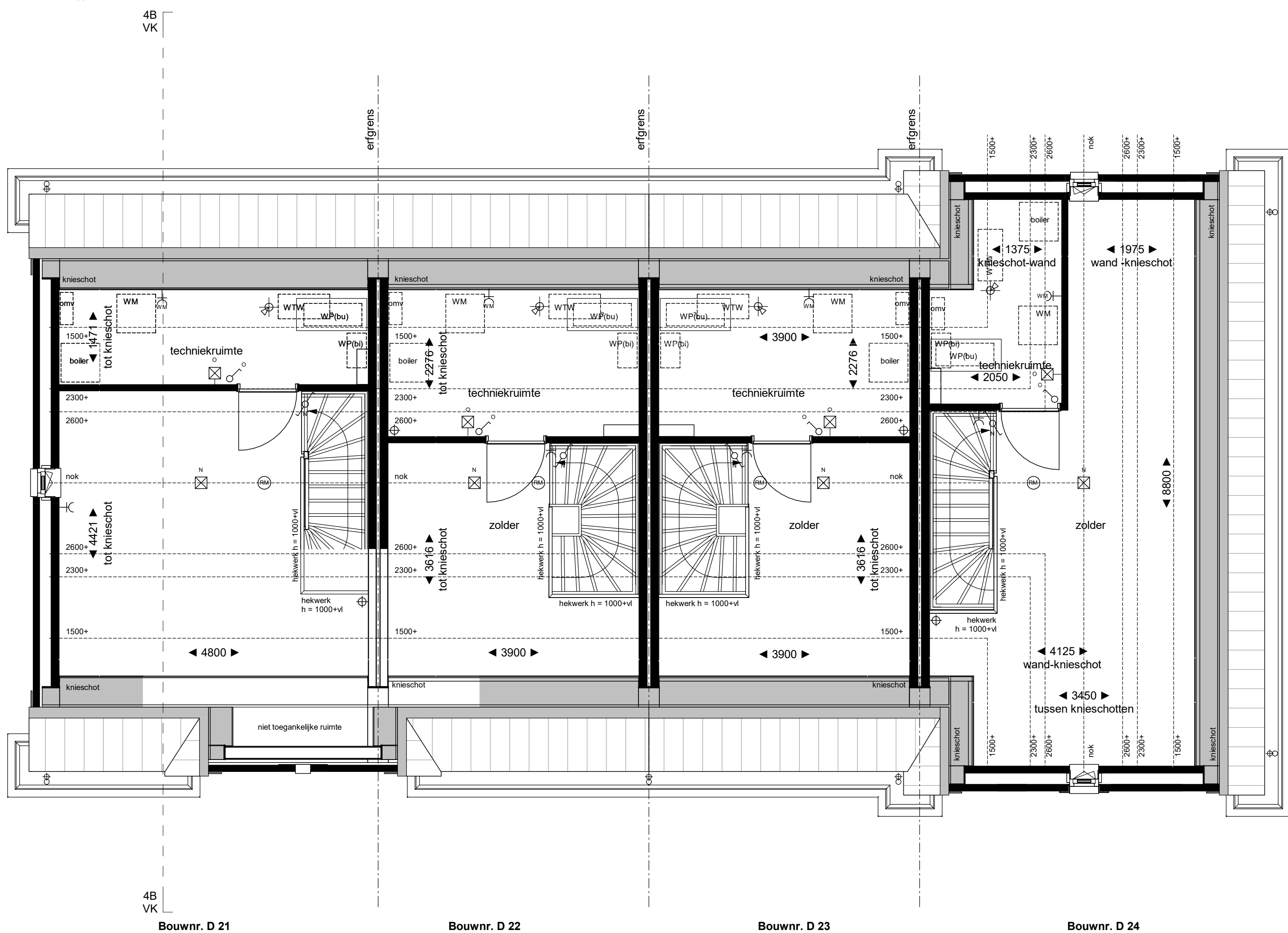
tweede verdieping 1:50
