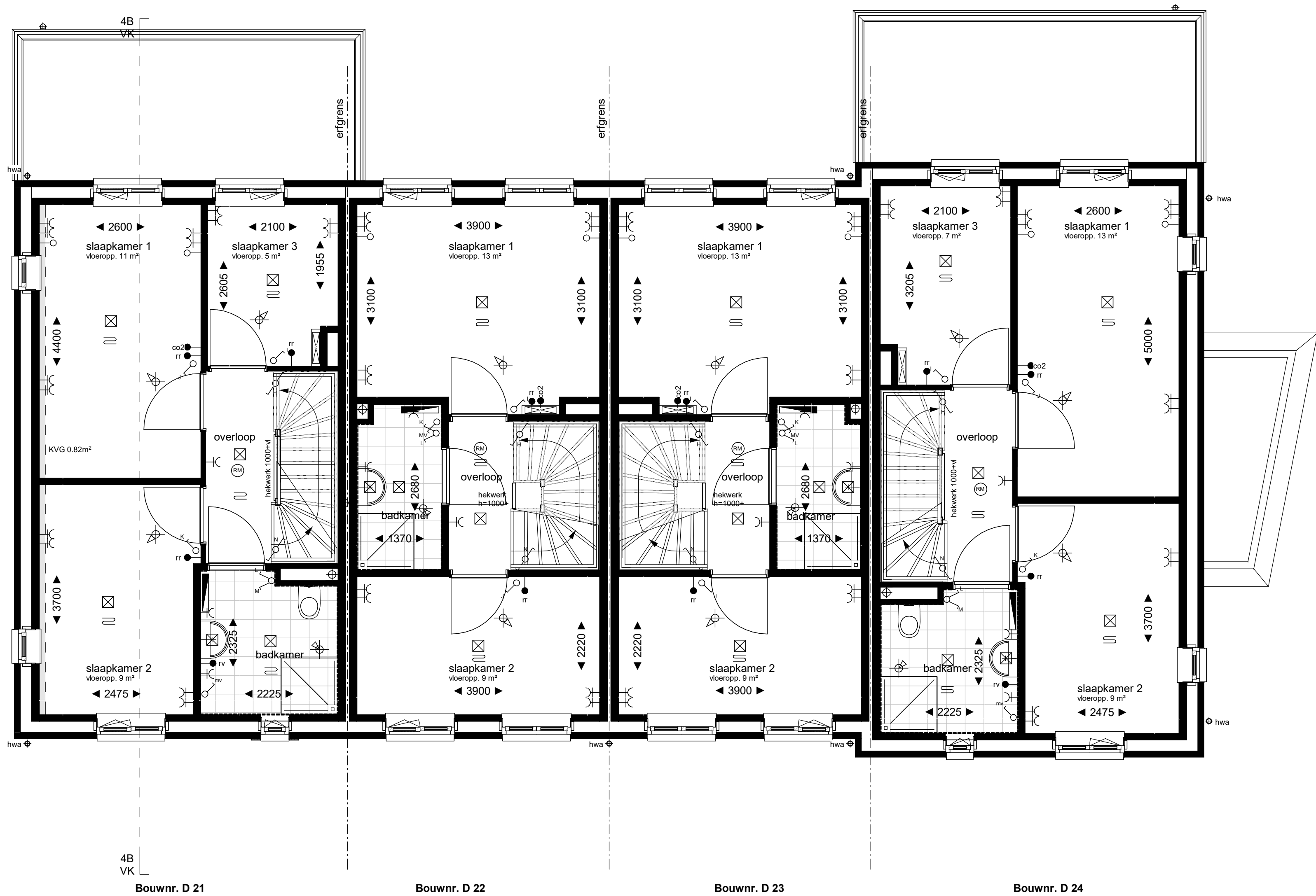
eerste verdieping 1:50
