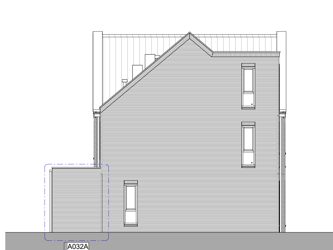
linker zijgevel 1 : 100
