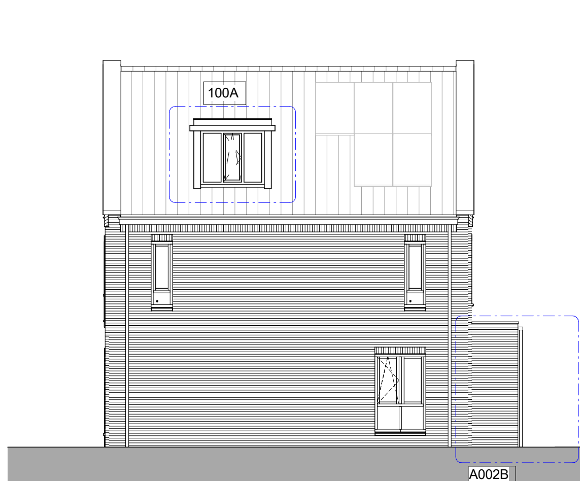
rechter zijgevel 1 : 100
