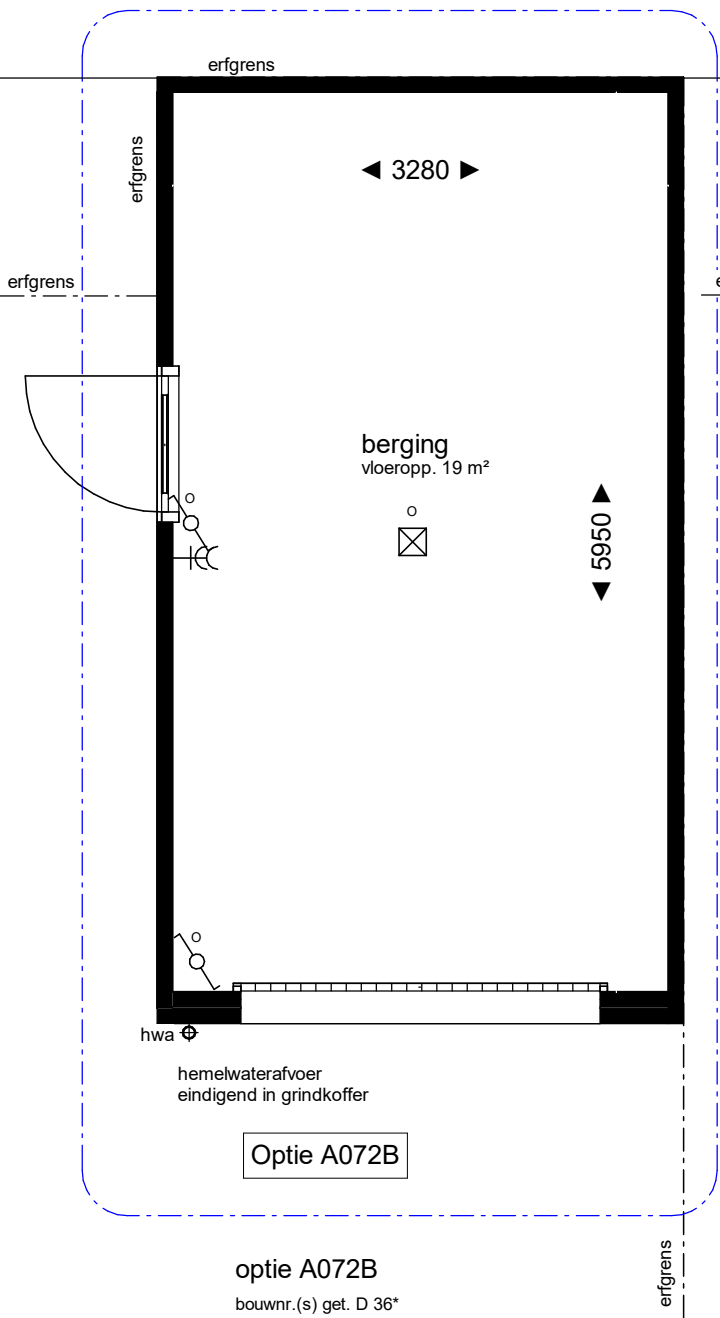
begane grond 1 : 50
