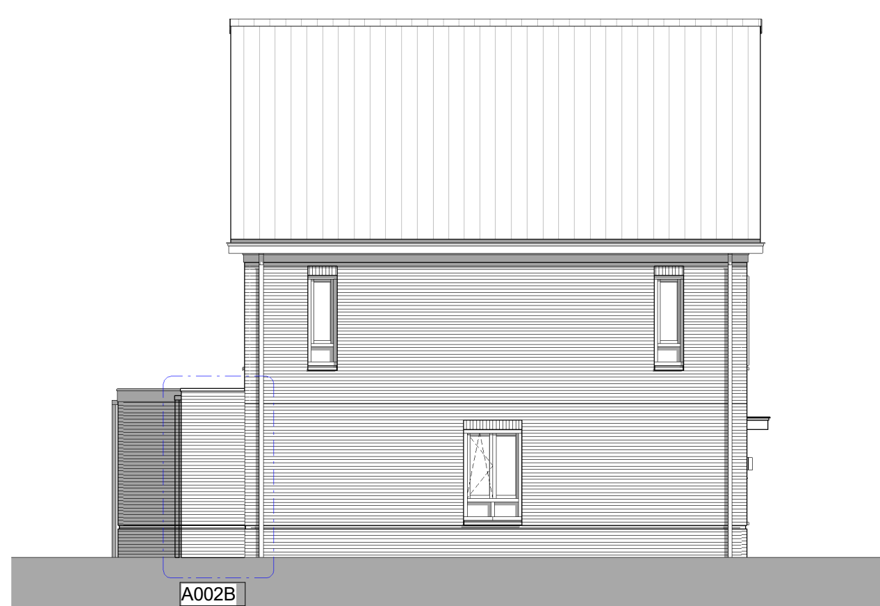
linker zijgevel 1 : 100
