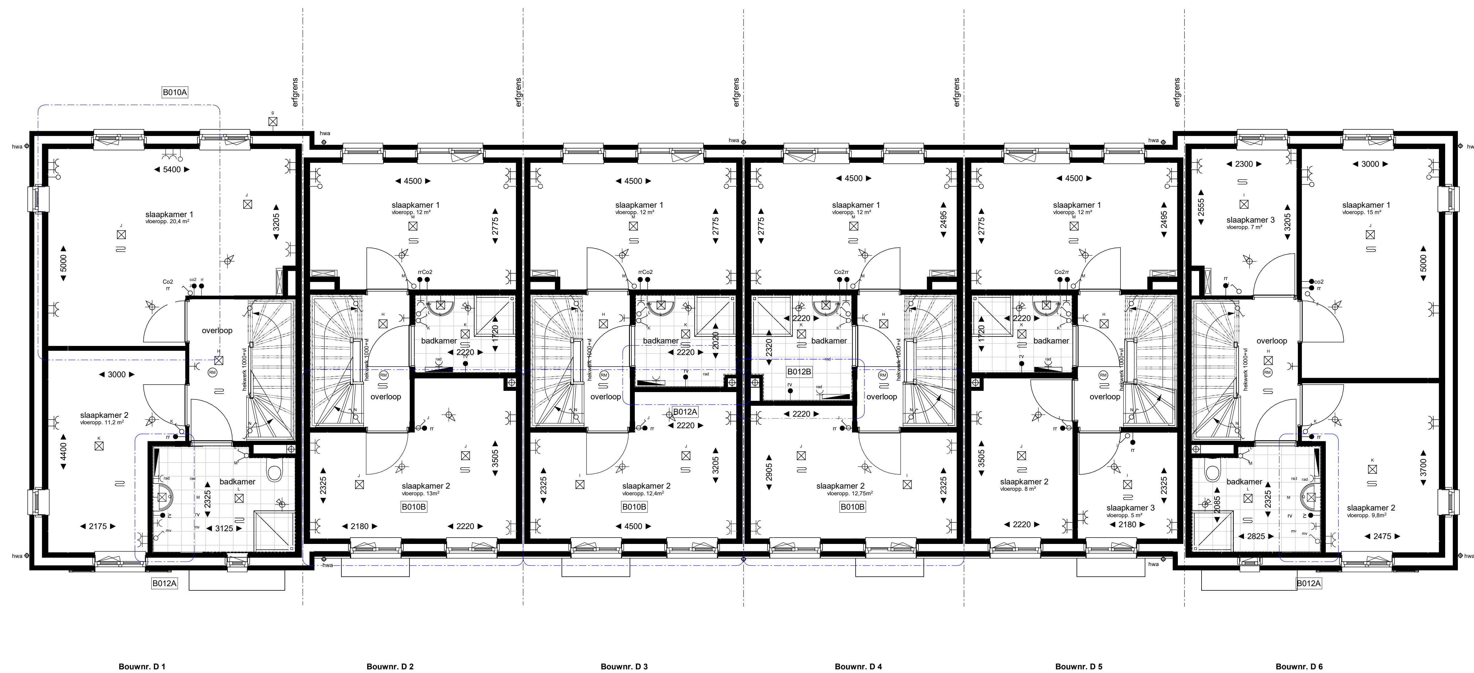
eerste verdieping 1 : 50
