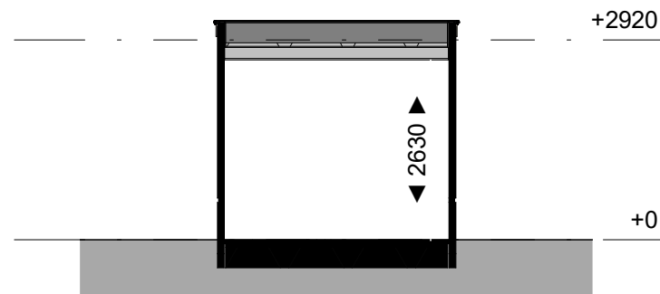
doorsnede A-A 1 : 100
