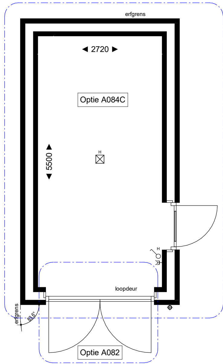
begane grond 1:50
